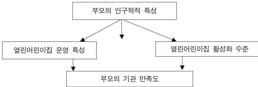
<그림 1> 연구모형
